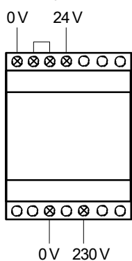
Fig. 1 Wiring for 24 V
