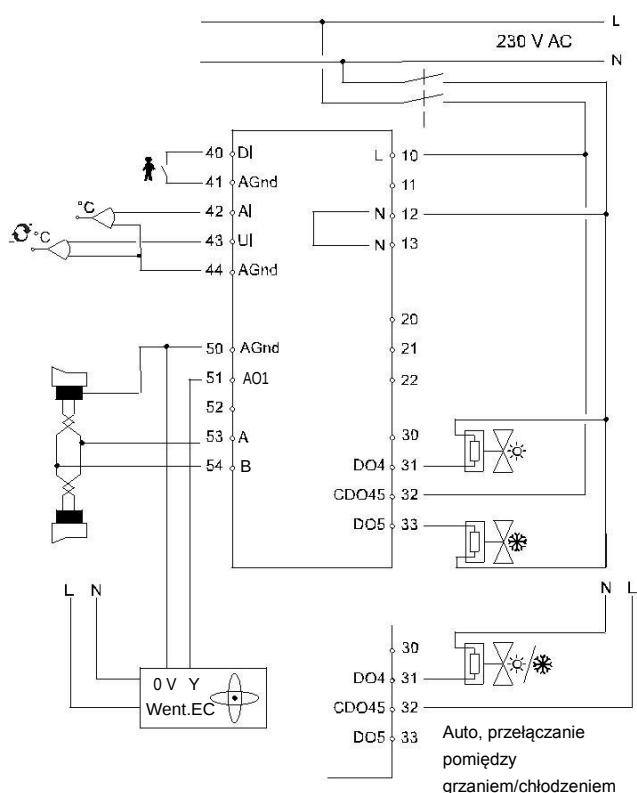
Schemat okablowania do podłączenia wentylatora do RCF-230 CTD
