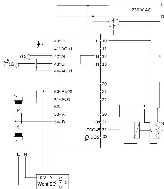
Schemat połączeń z grzałką elektryczną
