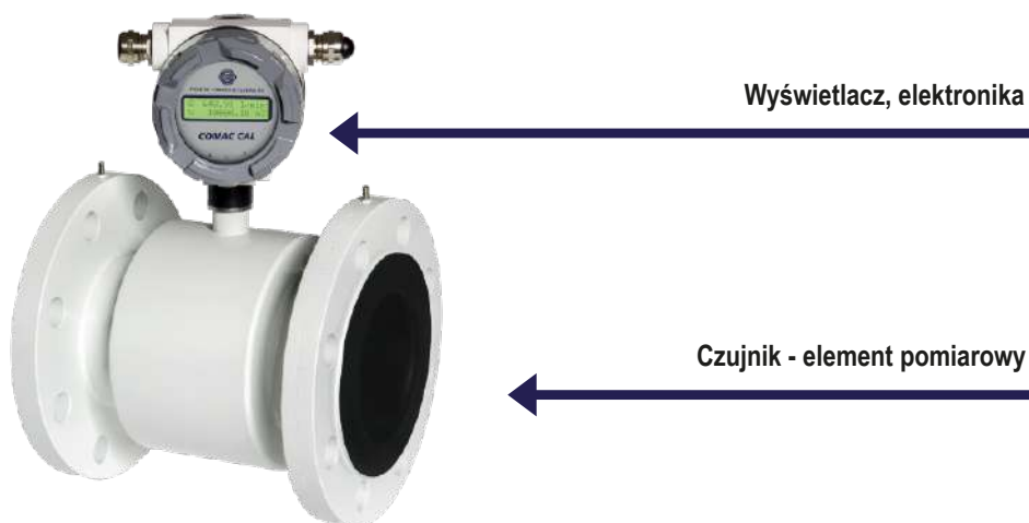
Zdjęcie 1. Budowa przepływomierza elektromagnetycznego
