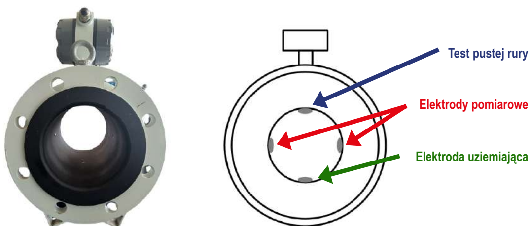
Zdjęcie 2. Wnętrze czujnika
