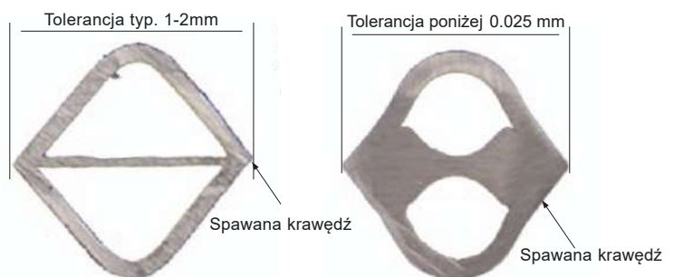
Zdjęcie 7. Porównanie profilu tradycyjnej rurki Pitota (z lewej) z profilem rurki Pitota w Deltaflow (z prawej)
